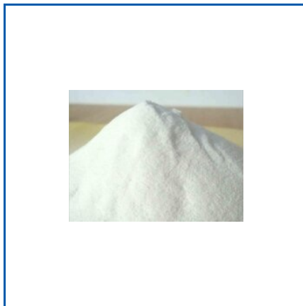
ZINC BROMIDE
